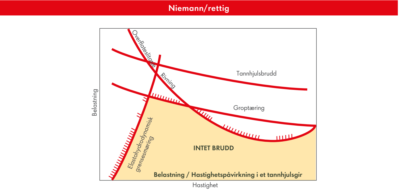
Koniske og sylindriske gir (DIN 51509)
